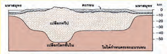
รูปที่ 7: เทือกเขาจะมีรากฝังลึกอยู่ที่พื้นดิน (Earth, Press และ Siever หน้า 413)
