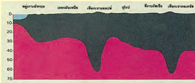
รูปที่ 8: ส่วนที่เป็นแผ่นผั่ง เทือกเขาที่มีรูปร่างเหมือนสลัก จะมีรากฝังแน่นอยู่ใต้พื้นดิน (Anatomy of the Earth ของ Cailleux หน้า 220)
