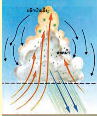
รูปที่ 20: เมฆฝนฟ้าคะนอง หลังจากที่ยกอนเมฆขยายตัวใหญ่ขึ้น น้ำฝนจึงกลั่นมาจากก้อนเมฆดังกล่าว (Weather and Climate ของ Bodin หน้า 123)
